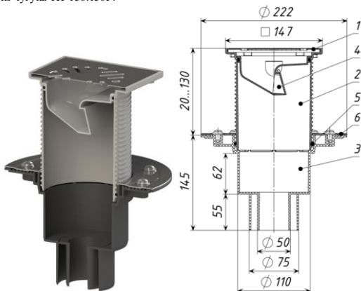
Рис. 1 ТП-310.1N Трап с незамерзающим запахозапирающим устройством
