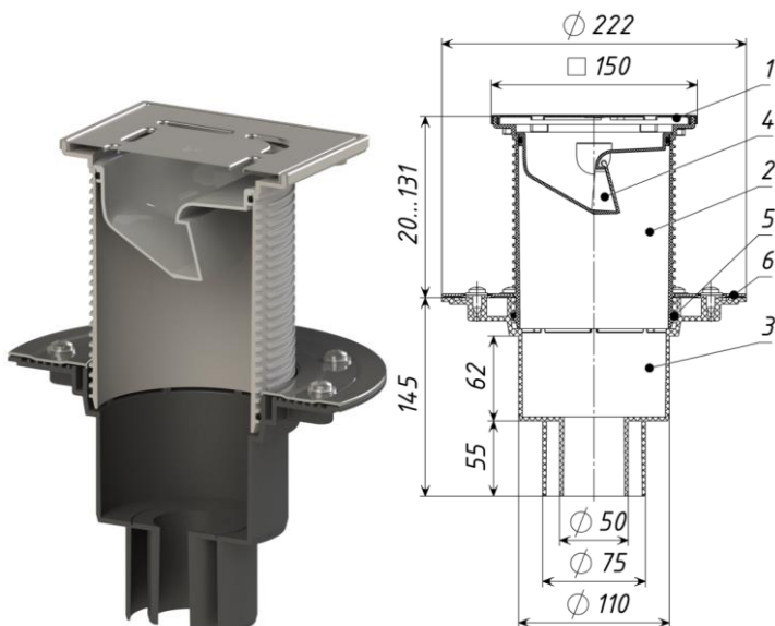
Рис. 1 ТП-310.1N-3000 Трап с незамерзающим запахозапирающим устройством
