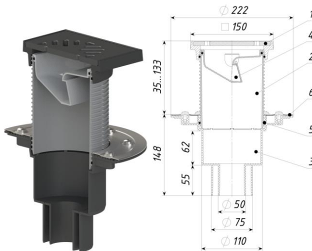
Рис. 1 ТП-310.1 PNG Трап с незамерзающим запахозапирающим устройством
