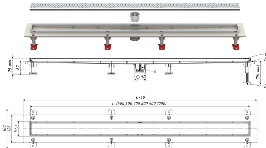
Рис. 1 – Габаритные размеры
