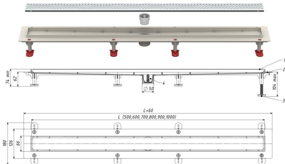
Рис. 1 – Габаритные размеры
