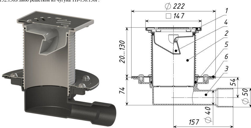
Рис. 1 ТП-510.1N Трап с незамерзающим запахозапирающим устройством
