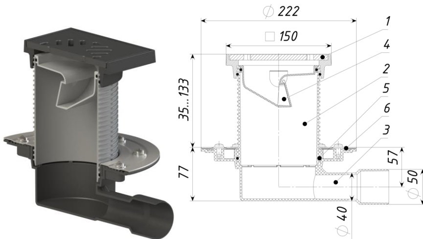
Рис. 1 ТП-510.1 PNG Трап с незамерзающим запахозапирающим устройством
