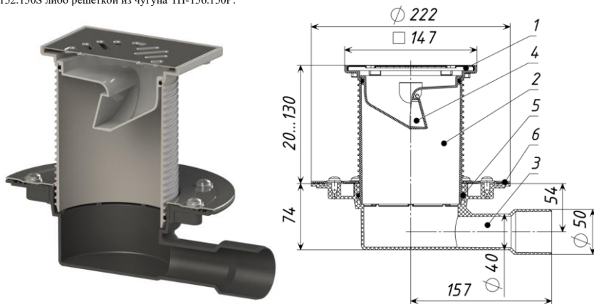
Рис. 1 ТП-510.1N Трап с незаморажающим запахозапирающим устройством
