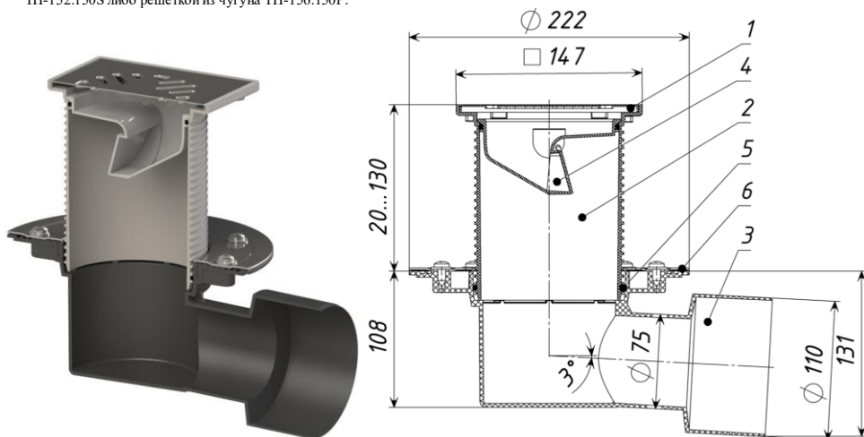
Рис. 1 ТП-5100.1N Трап с незамерзающим запахозапирающим устройством
