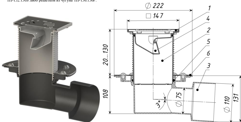
Рис. 1 ТП-5100.1N Трап с незамёрзающим запахозапирающим устройством
