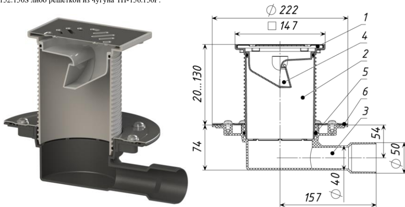
Рис. 1 ТП-510.1N Трап с незамerзающим запахозапирающим устройством
