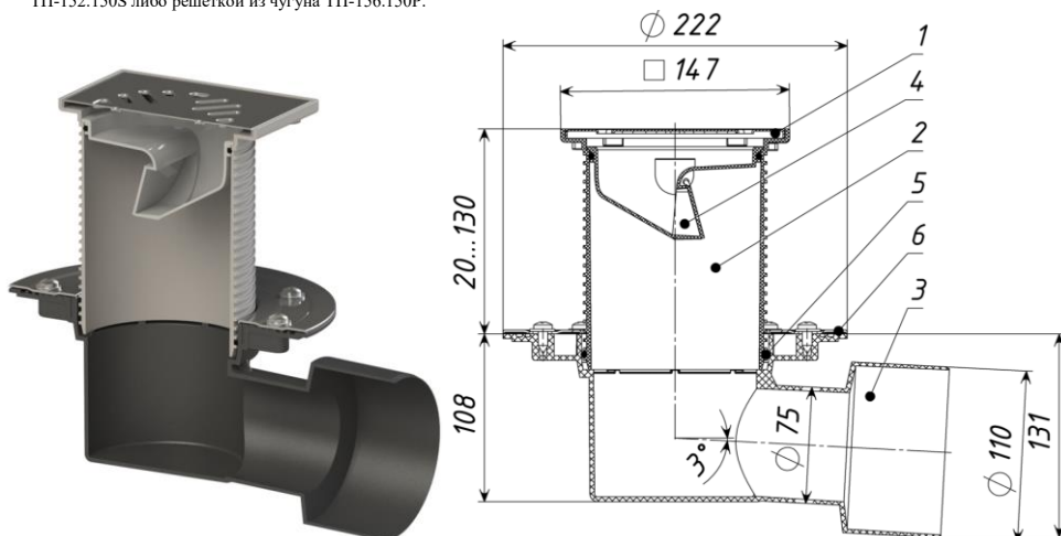
Рис. 1 ТП-5100.1N Трап с незаморажающим запахозапирающим устройством
