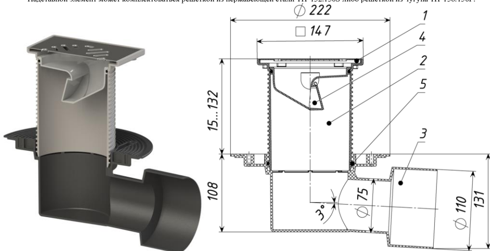
Рис. 1 ТП-5100N Трап с незамерзающим запахозапирающим устройством
