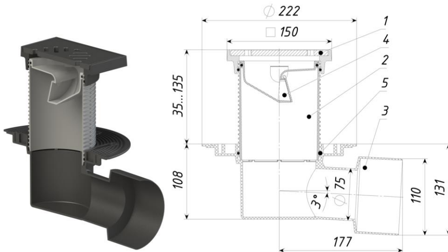
Рис. 1 ТПИ-5100 PNG Трап с незамерзающим запахозапирающим устройством
