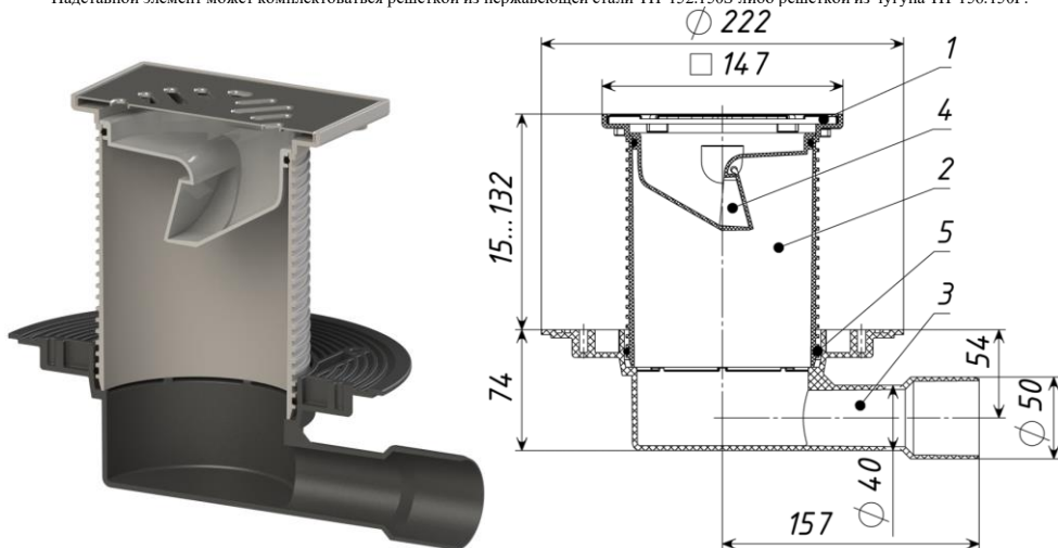
Рис. 1 ТП-510N Трап с незамерзающим запахозапирающим устройством
