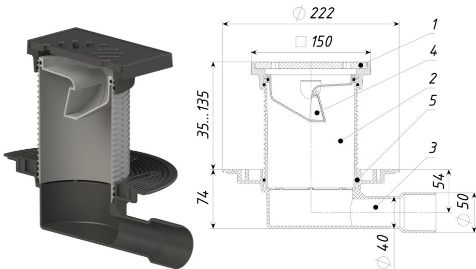
Рис. 1 ТПИ-510 PNG Трап с незамерзающим запахозапирающим устройством
