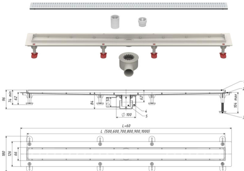
Рис. 1 – Габаритные размеры
