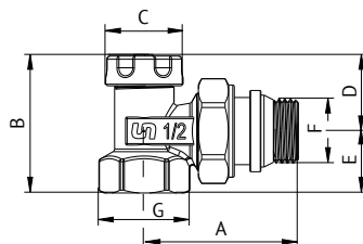
Вентиль обратный угловой НВ с разъёмным соединением быстрого монтажа
