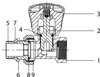
Вентиль ручной НВ с разъёмным соединением
