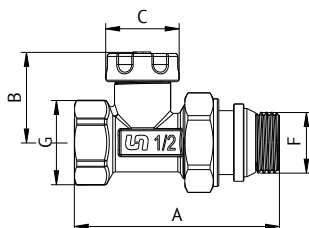
Вентиль обратный НВ с разъёмным соединением быстрого монтажа
