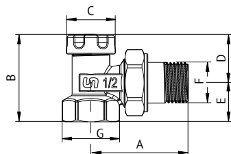
Вентиль обратный угловой НВ с разъёмным соединением
