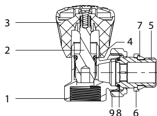
Вентиль ручной угловой НВ с разъёмным соединением
