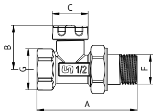
Вентиль обратный НВ с разъёмным соединением
