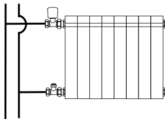
Двухтрубная система
