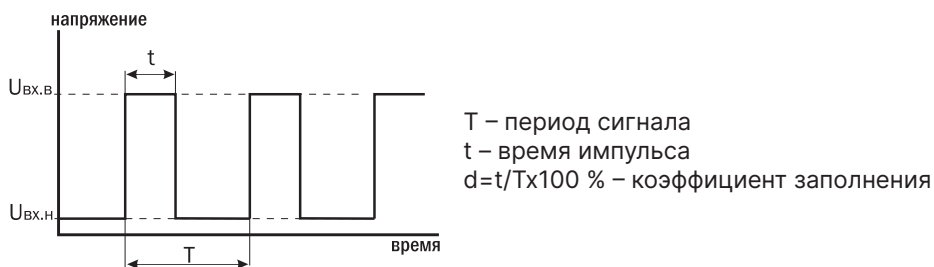
Рис.10 Характеристики ШИМ-сигнала
