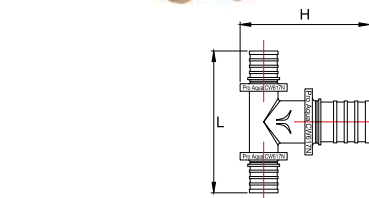
Тройник переходной
