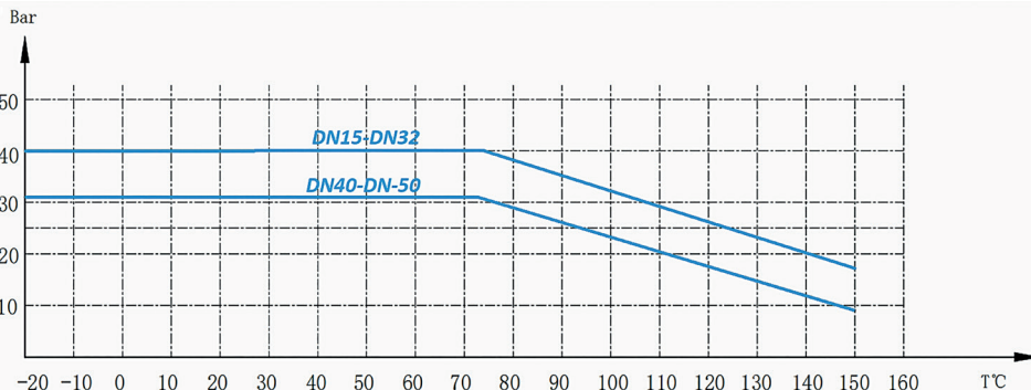
рис. 1. Зависимость рабочего давления от температуры перемещаемой среды
