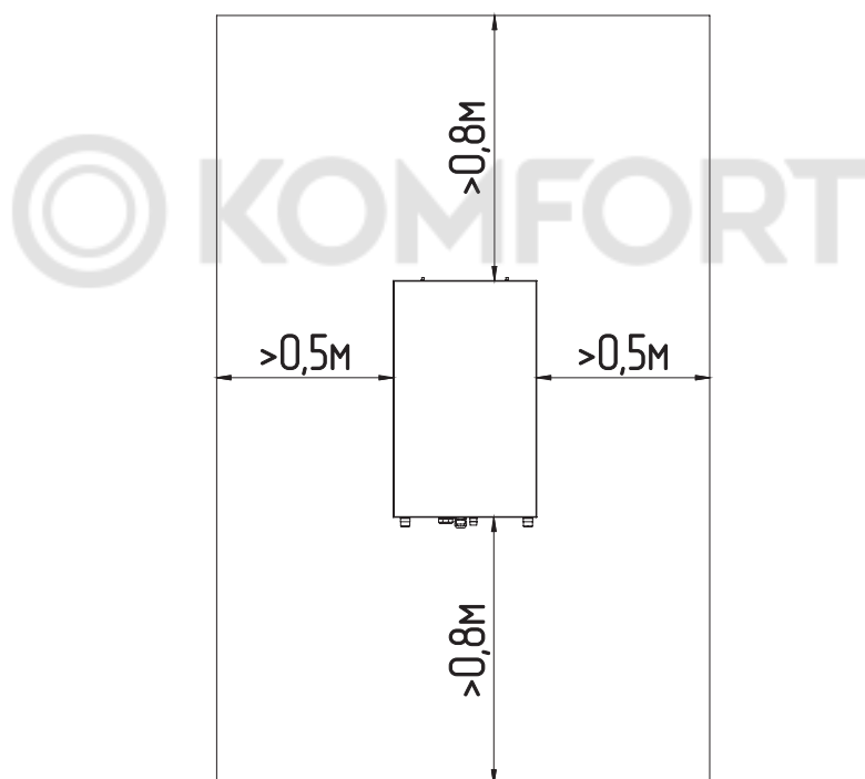
Рис.4 Схема размещения котла в котельной
