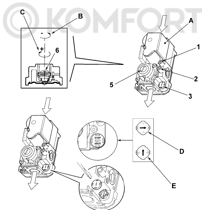
рис. 19 - Переналадка котла на другой вид газа
