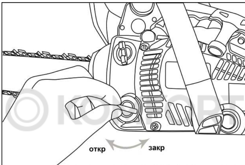
Рис. 12. Открывание горловины масляного бака
