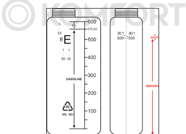
Рис. 11. Емкость для приготовления топливной смеси
