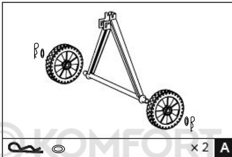
Рис. 3 Установка колес
