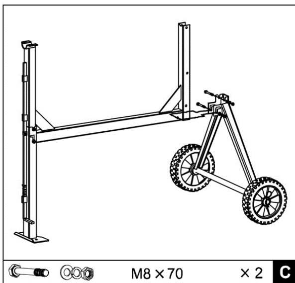
Рис. 4 Установка стойки
