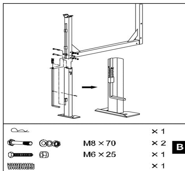
Рис. 5 Сборка рамы
