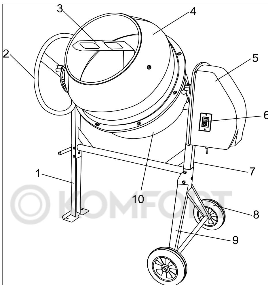
Рис. 2. Общий вид
