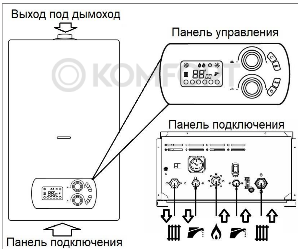
Рис. 1. Общий вид газового котла
