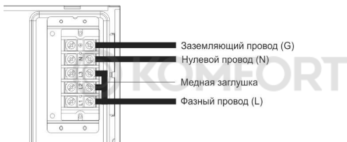
Рис 11. Однофазное подключение прибора
