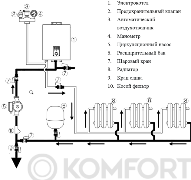
Рис. 3. Схема подключения в систему с радиаторным отоплением.
