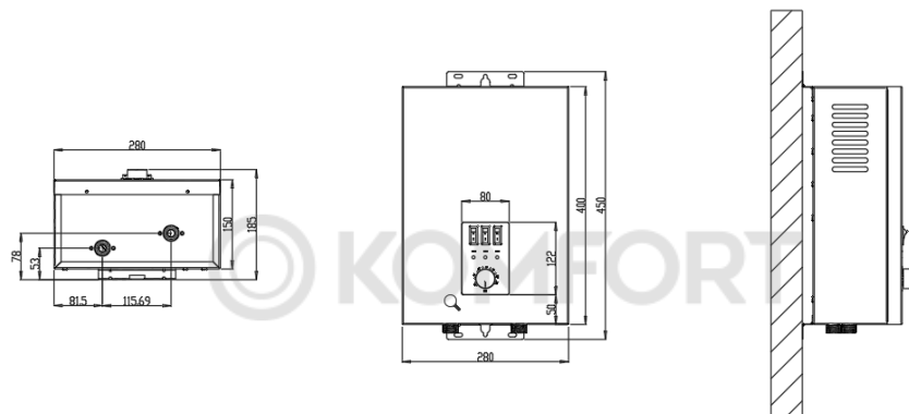
Рис. 7. Монтажные размеры
