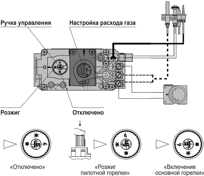
Рисунок 10 Элементы управления и регулировки на газовом блоке
