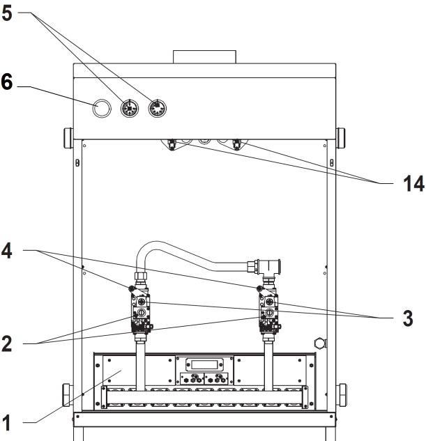
Рисунок 3 Особенности котла ТОРИНО-100 с двумя газовыми блоками 820 NOVA mV
