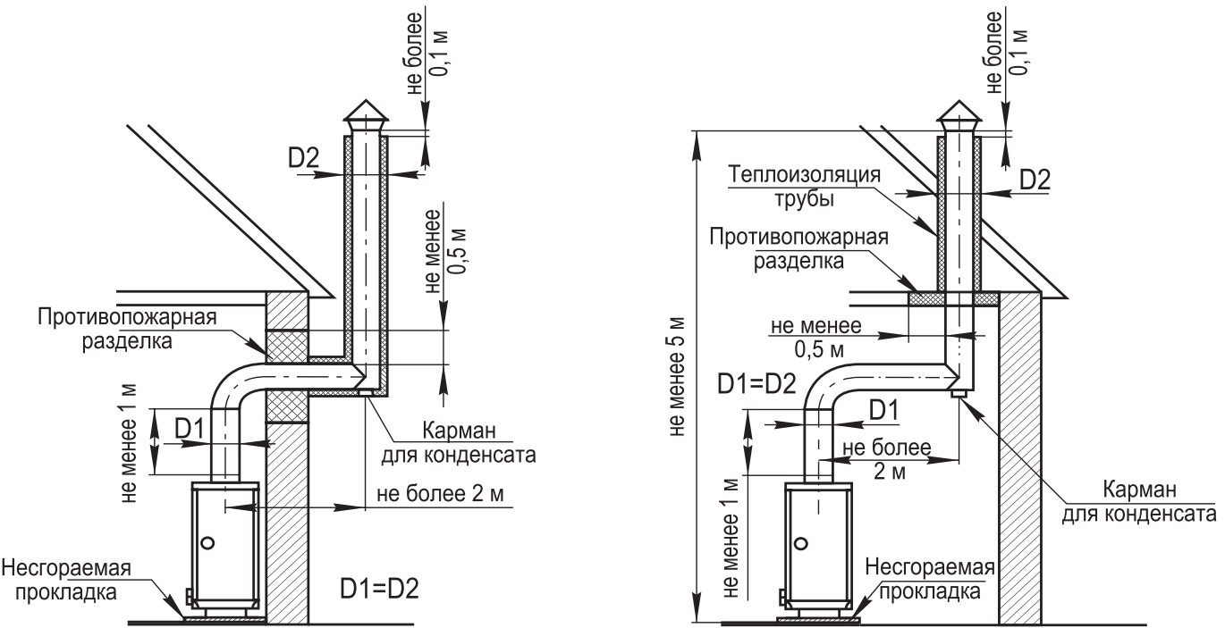
Рисунок 7 Схема установки дымовой трубы с выводом через стену и с выводом через потолочное перекрытие.
