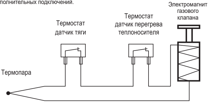
Рис. 4. Электрическая схема котла
