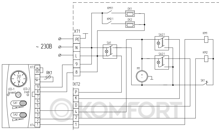
Рисунок 11. Принципиальная схема занавесы KVC-A08E3-12 с пультом управления KRC-32
