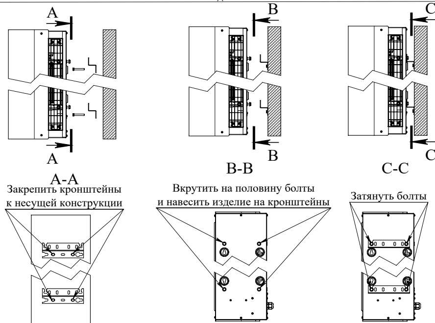
Рисунок 14. Схема крепления занавесы вертикально к стене с помощью кронштейнов.
