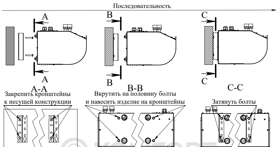
Рисунок 13. Схема крепления занавес горизонтально над проемом к стене с помощью кронштейнов.
