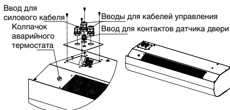
Рисунок 3. Воздушно-тепловая завеса.
