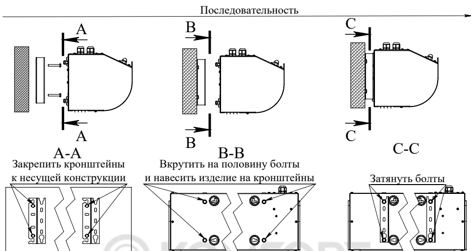
Рисунок 13. Схема крепления занавеси горизонтально над проемом к стене с помощью кронштейнов.
