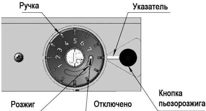
Рис. 10. Элементы управления на газовом блоке управления TGV307
