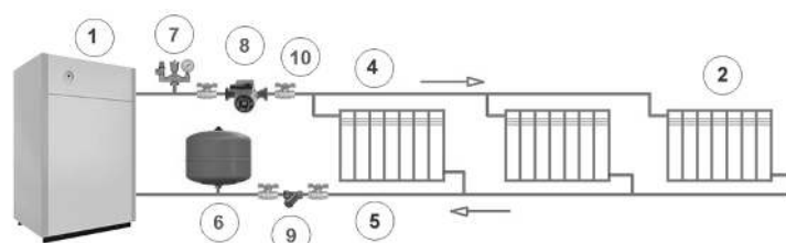
Рис. 8. Закрытая система отопления
