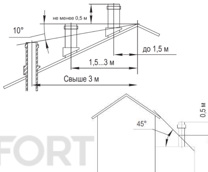
рис. 6 – Схема расположение дымовой трубы
