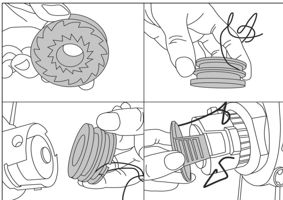
Рис. 10. Намотка лески
