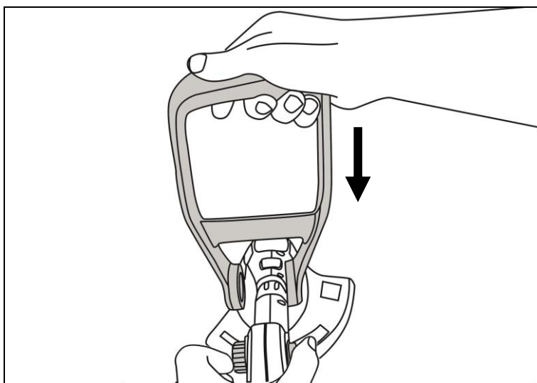
Рис. 3. Установка рукоятки
