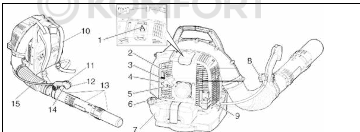
Рис. 1 Общий вид
