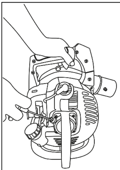
Рис. 12 Запуск двигателя
