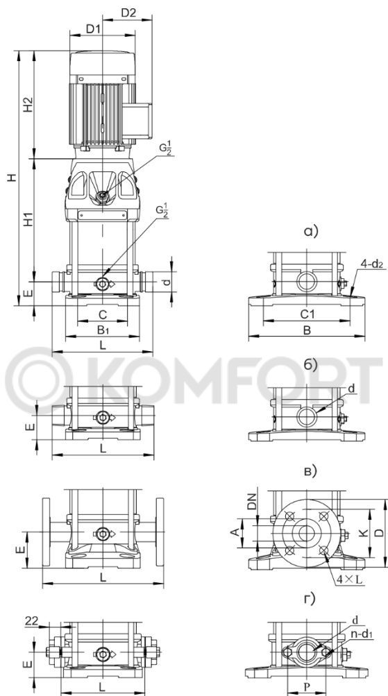
Рисунок 8 - Габаритно-присоединительные размеры CDM/CDMF а) vactaulic (групплок); б) трубная резьба; в) DIN-фланец; г) овальный фланец
