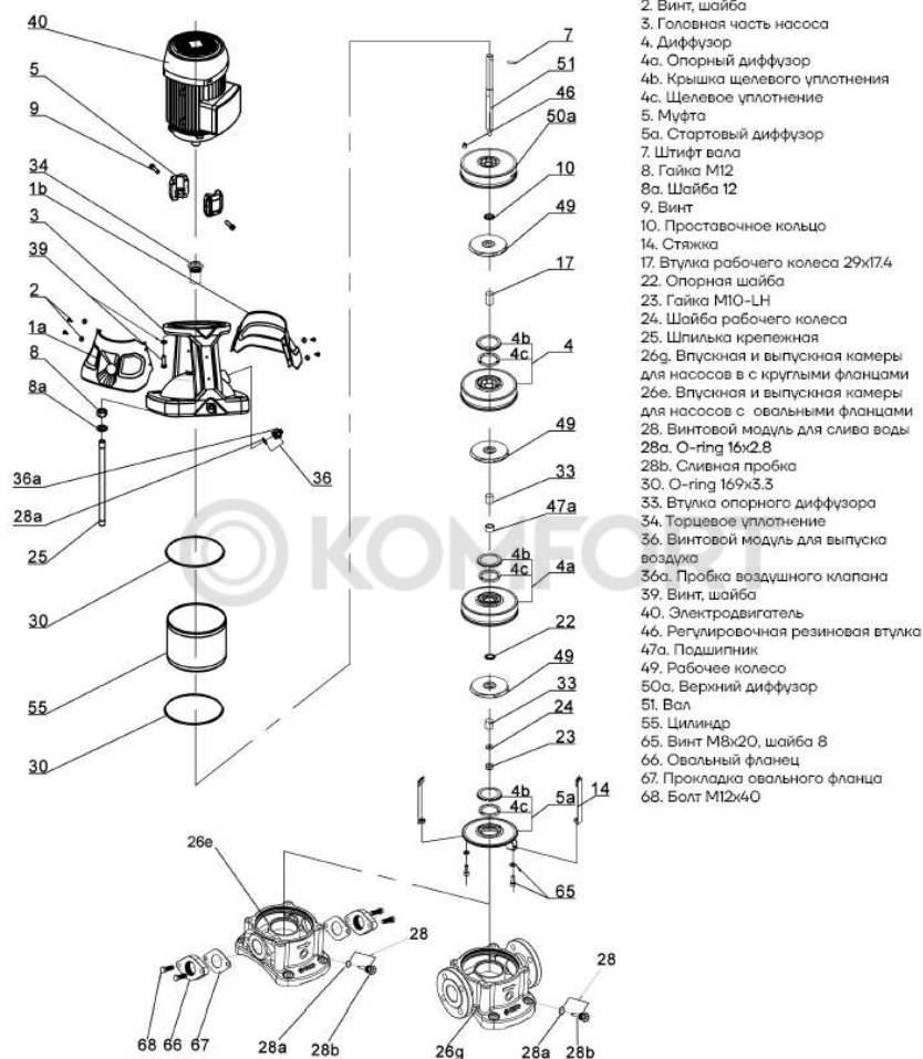
Рисунки 7-F CDM 10
