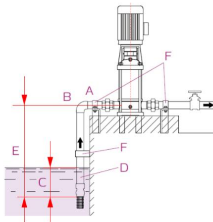
Рис. 6 Правильная установка
