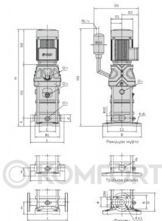
Рисунок 9 - Габаритно-присоединительные размеры высокотемпературных (до +180°C) насосов CDMF
