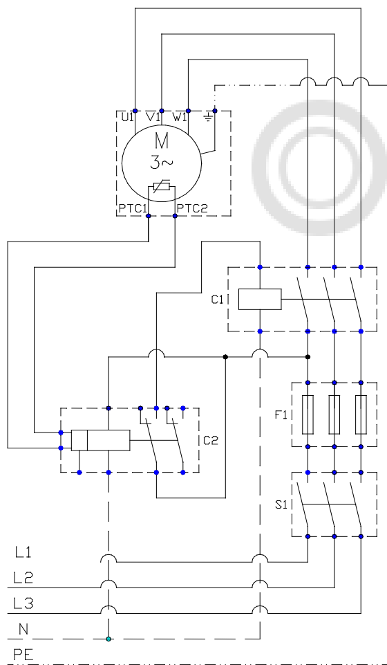
Трехфазный электродвигатель со встроенным терморезистором (PTC)
