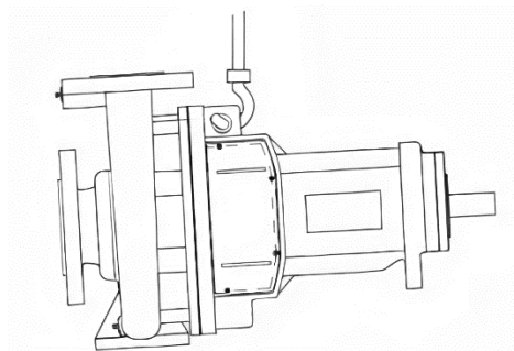
Рис. 5 Правильный способ строповки насоса без двигателя
