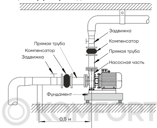
Рис. 12 Схема подключения насоса
