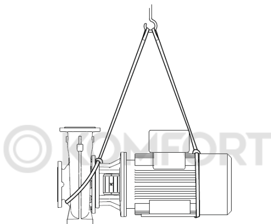
Рис. 3 Правильный способ строповки насоса без плиты-основания
