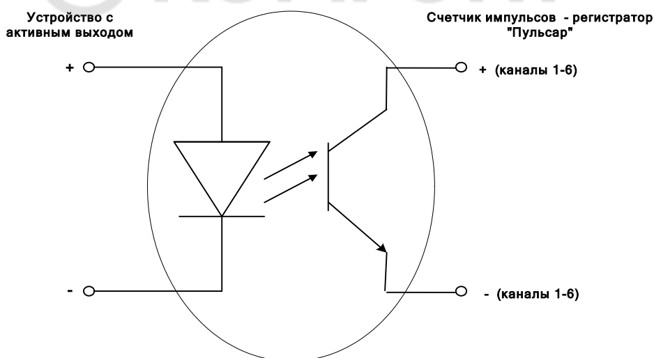
Рис. 7.1 Схема подключения устройств с активным выходом
