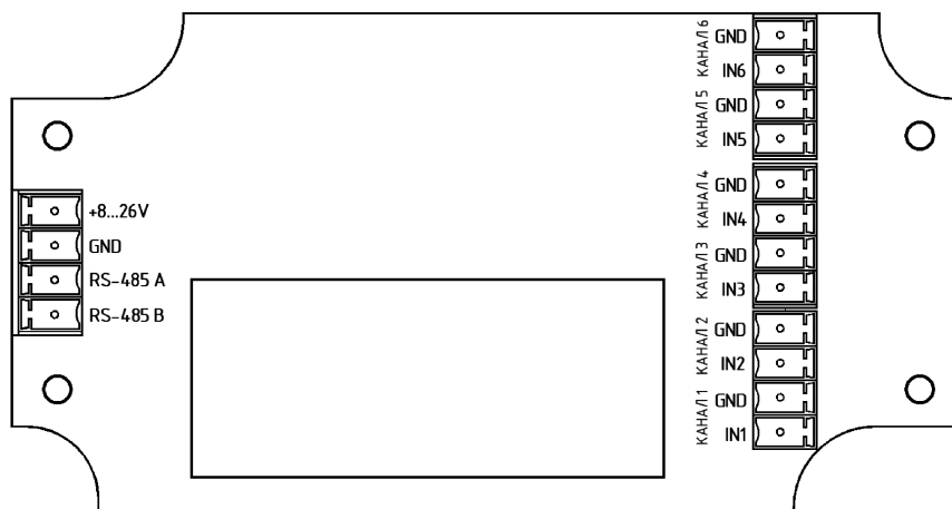
Рис. 7.2 Схема клеммников платы
