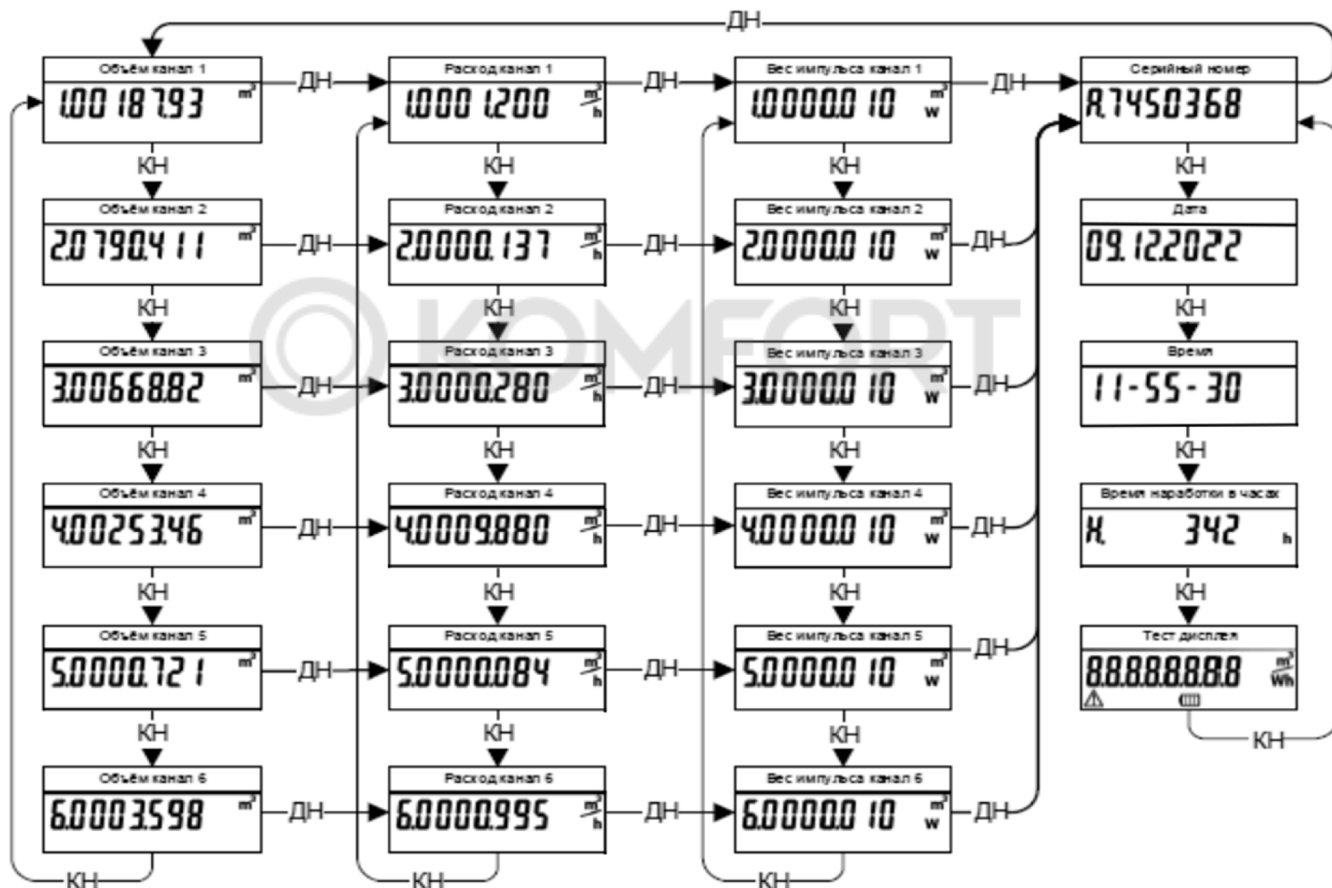
Рис. 4.1 Схема меню
