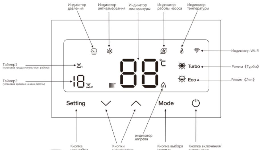
Рис. 3. Панель управления
