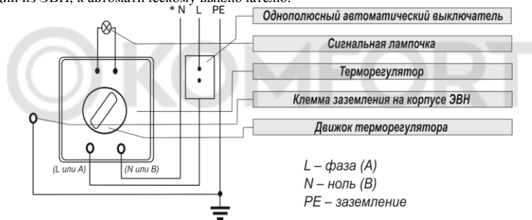
Рис. 7. Схема электрическая для моделей E-Series, O'Pro, EGO, O'Pro +
