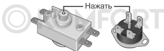
Рисунок 2. Схема расположения кнопки термовыключателя
