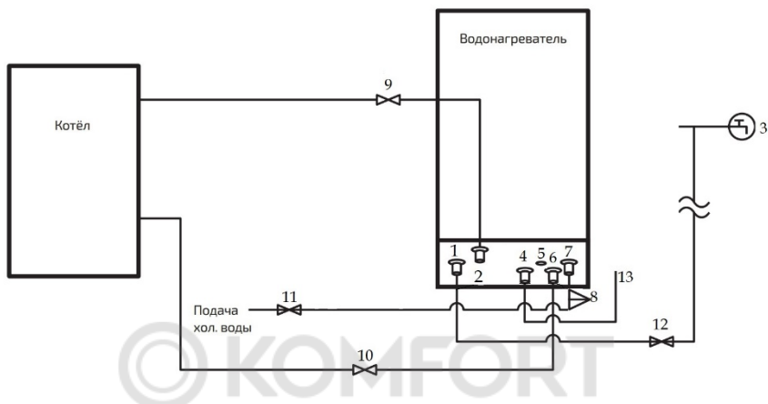
Рисунок 2. Подключение КЭВН
