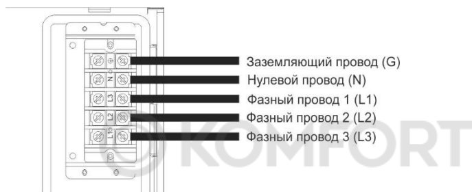
Рис 12. Трехфазное подключение прибора
