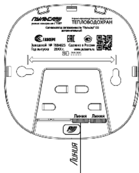
Сигнализатор загазованности "Пульсар" СО дополнительный
