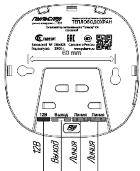
Сигнализатор загазованности "Пульсар" СН основной
