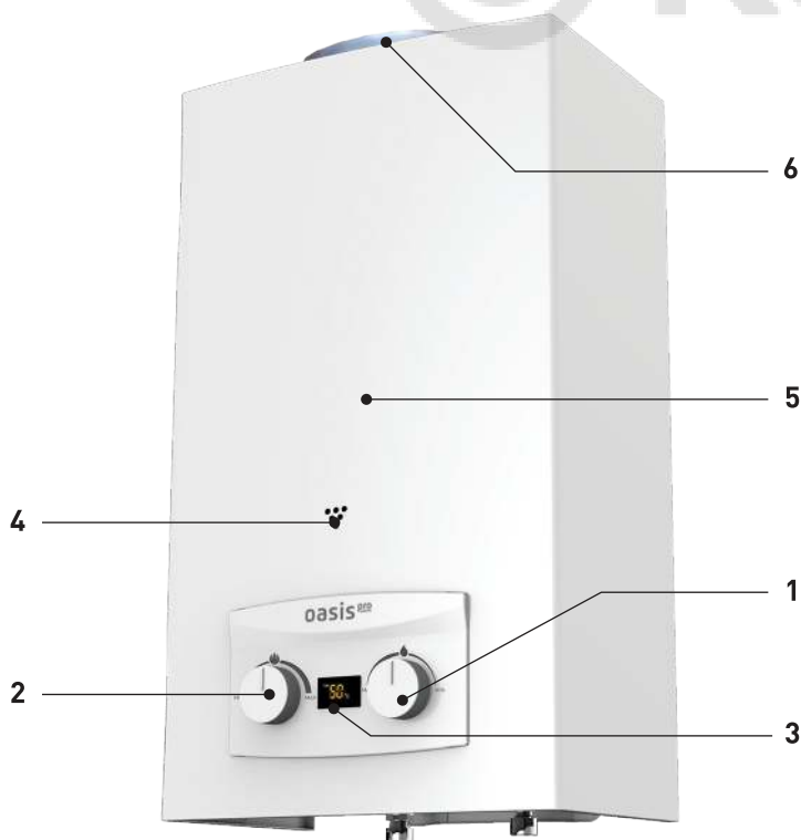
Рис. 1. Аппарат водонагревательный проточный газовый бытовой oasis pro 1 - ручка водяного регулятора; 2 - ручка газового регулятора; 3 - цифровой индикатор температуры горячей воды; 4 - окно смотровое; 5 - облицовка; 6 - патрубок дымоотвода.
