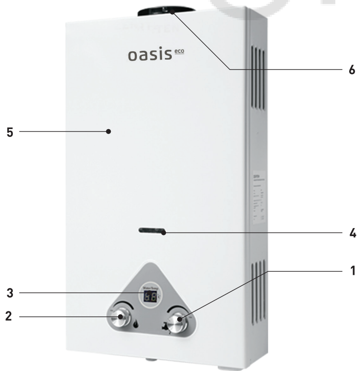
Рис. 1. Аппарат водонагревательный проточный газовый бытовой Oasis Eco 1 - ручка водяного регулятора; 2 - ручка газового регулятора; 3 - цифровой индикатор температуры горячей воды; 4 - окно смотровое; 5 - облицовка; 6 - патрубок дымоотвода.
