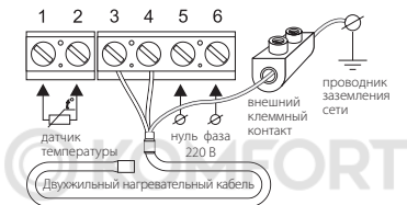
Схема подключения к 3-х проводной электрической сети
